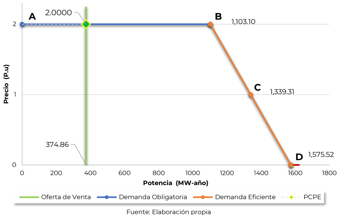
Fig. 12. Curvas de Demanda y Venta de Potencia BCA
