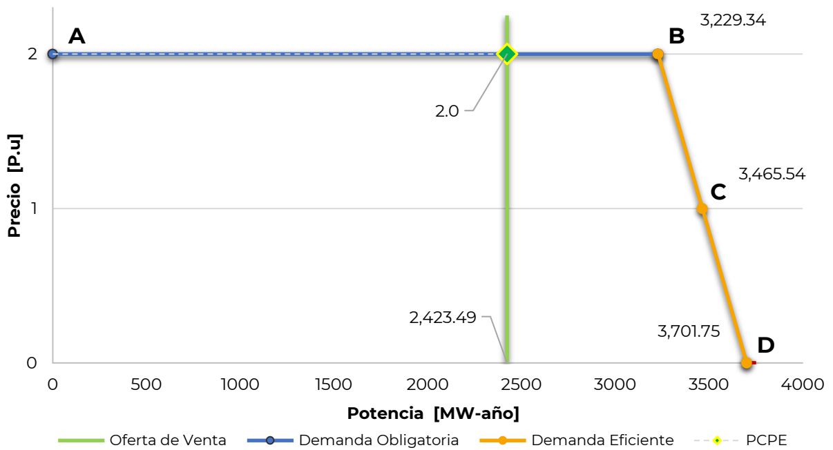
Fig. 9. Curvas de Demanda y Venta Estimadas BCA
