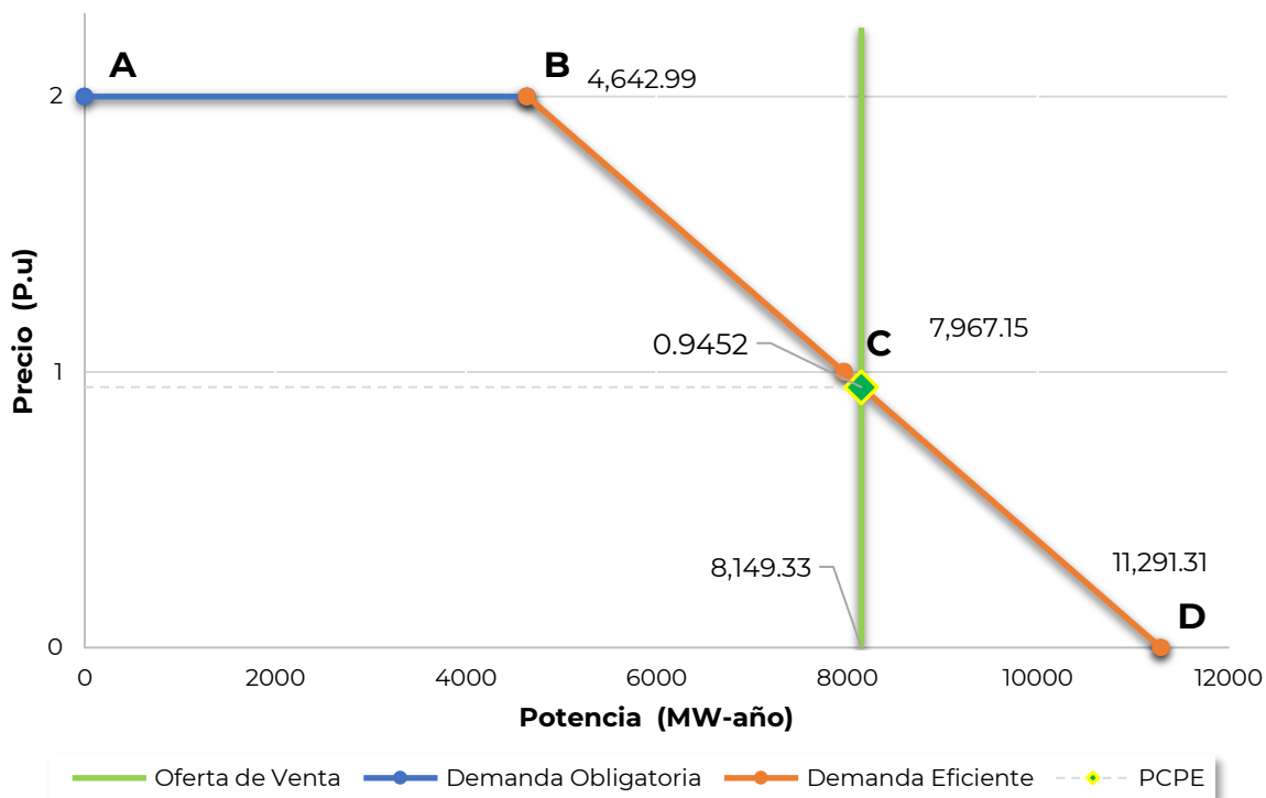
Fig. 13. Curvas de Demanda y Venta de Potencia SIN
